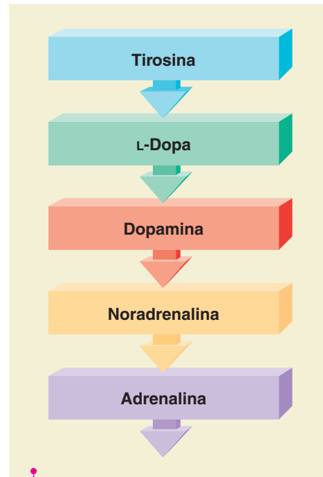
FIGURA 4.14 Pasos en la síntesis de catecolaminas a partir de la tirosina.
