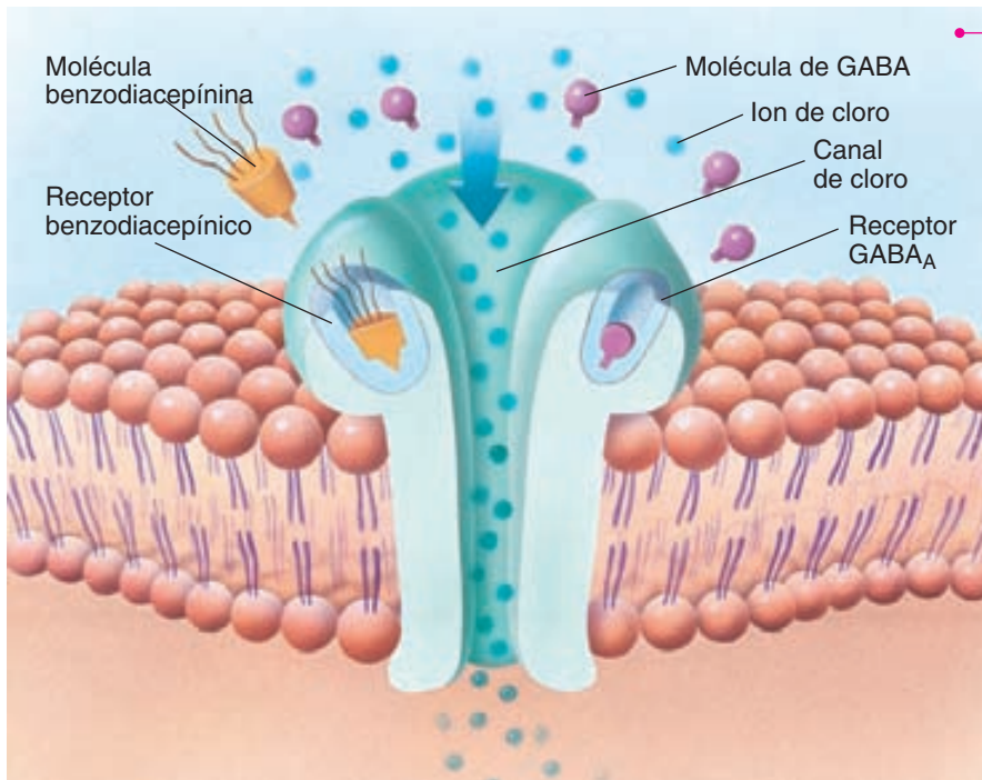
FIGURA 4.18 El complejo receptor benzodiacepínico GABA A .
