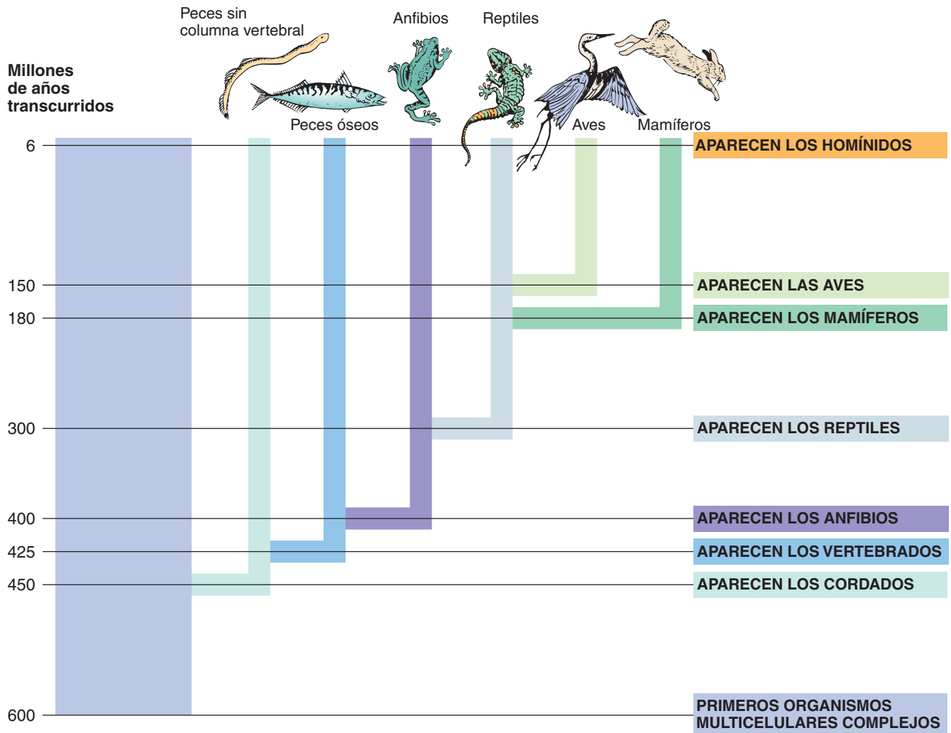
FIGURA 2.10 Evolución de los vertebrados.
