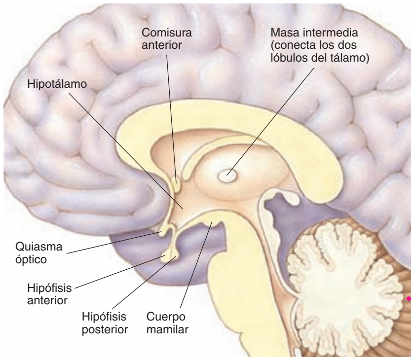
FIGURA 13.2 Vista de la línea media de la hipófisis posterior y anterior y estructuras adyacentes.
