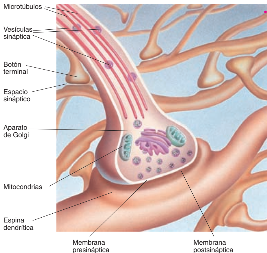
FIGURA 4.7 Anatomía de una sinapsis típica.
