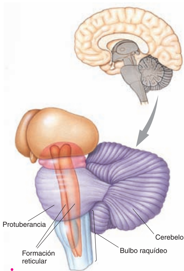
FIGURA 3.21 Estructuras del mielencéfalo (bulbo raquídeo) y del metencéfalo humanos.
