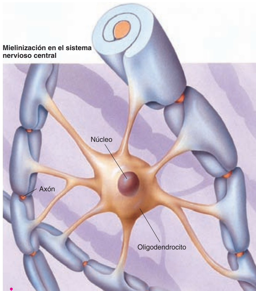
FIGURA 3.9 Mielinización de los axones del SNC por un oligodendrocito y mielinización de los axones del SNP por células de Schwann.
