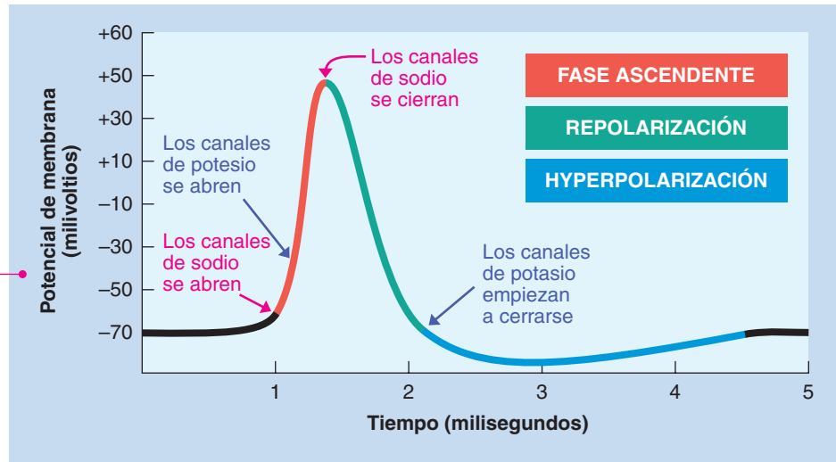
FIGURA 4.6 La apertura y el cierre de los canales controlados por voltaje de sodio y de potasio durante las tres fases del potencial de acción: fase ascendente, repolarización e hiperpolarización.
