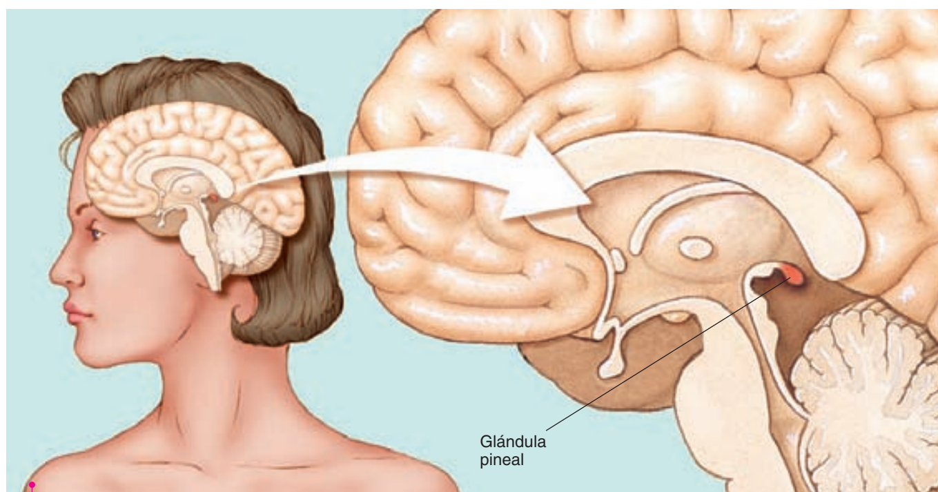
FIGURA 14.13 Localización de la glándula pineal, la fuente de melatonina.
